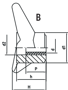
VERSIONE BOCCOLA OTTONE PASSANTE
