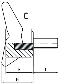
VERSIONE PERNO
