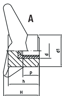
VERSIONE BOCCOLA OTTONE
